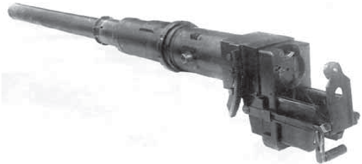
ՀՄՍ 1-ի 2Ա28 կիսաավտոմատ «Գրադ» հրանոթը գոյամարտի առաջին փուլում սպառազինության խիստ կարիք զգացող ինքնապաշտպանական ուժերի փոքրաթիվ «հզոր» կրակային միջոցներից էր:
